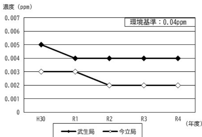
図 2-2-2 二酸化窒素の年平均値の推移
