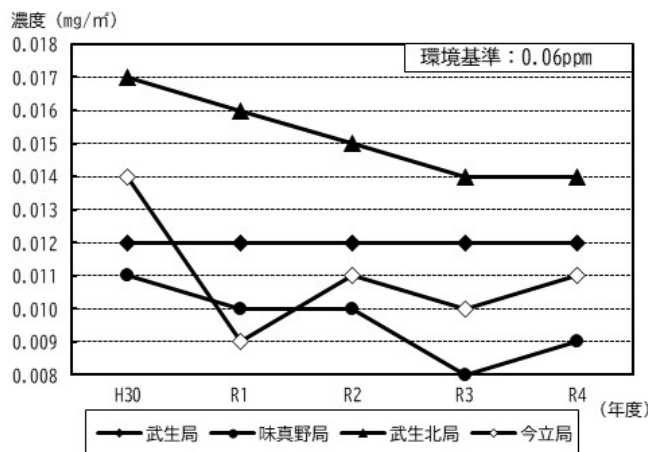
図 2-2-3 SPM の年平均値の推移
