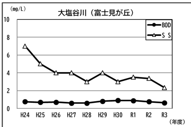
図 3-2-1 河川水質調査経年変化グラフ（生活環境項目）
