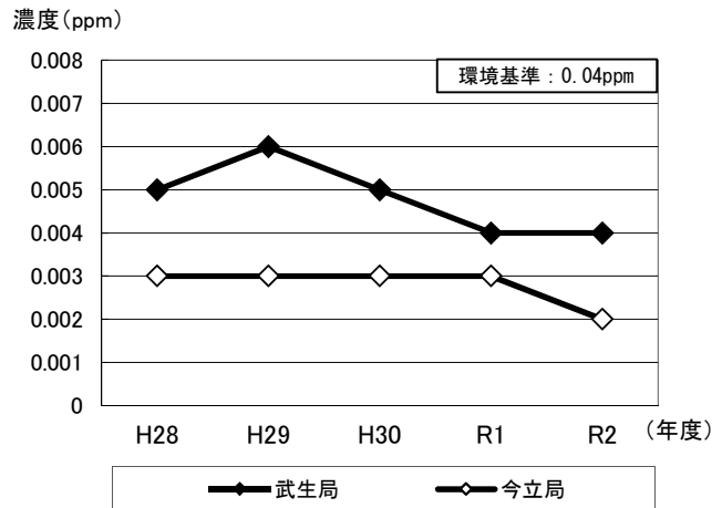
図 2-2-2 二酸化窒素の年平均値の変化
