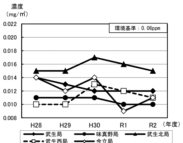
図 2-2-3 SPM の年平均値の推移
