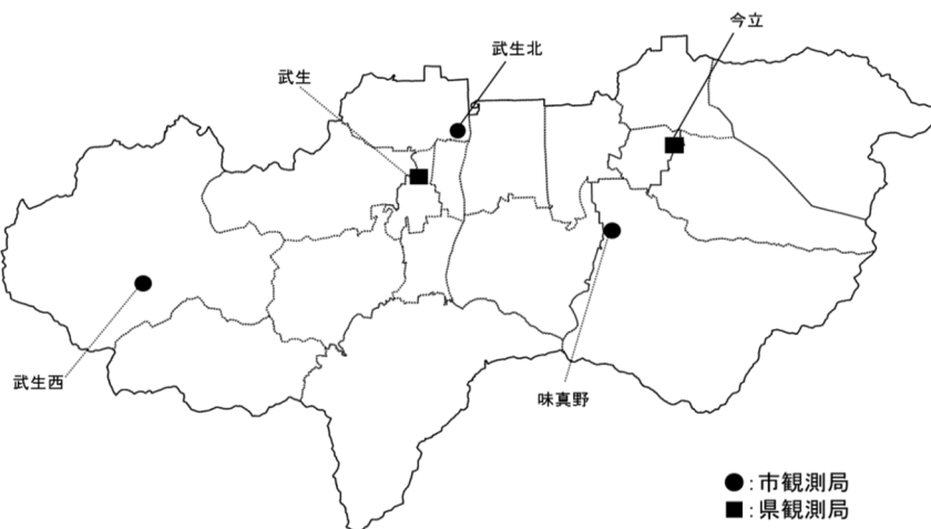
図 2-1 越前市内の大気汚染常時観測局の位置
