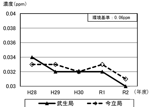
図 2-2-4 光化学オキシダントの年平均値の推移 (昼間 1 時間値)
