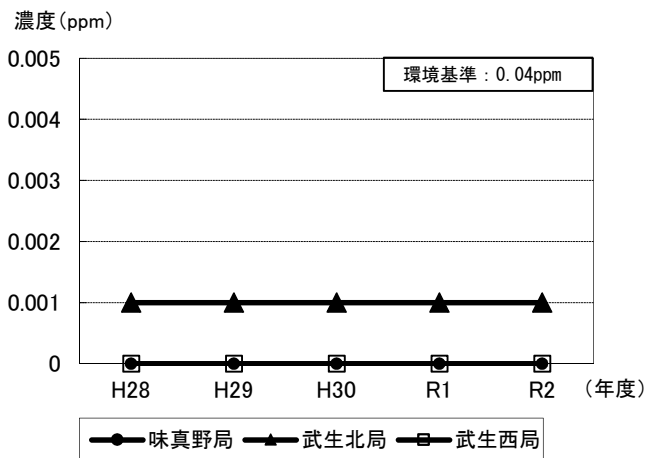
図 2-2-1 二酸化硫黄の年平均値の推移
