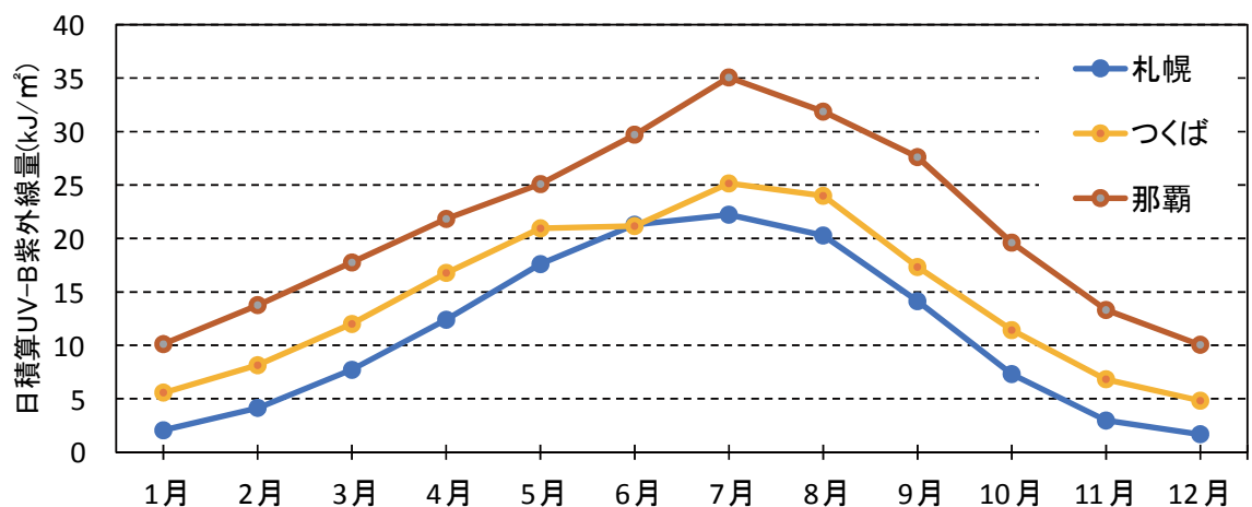
<図1-6 月別紫外線照射量( \text{kJ}/\text{m}^2 /日)>
